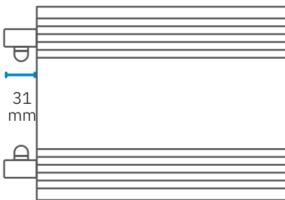
Vorstehende Anschlüsse
