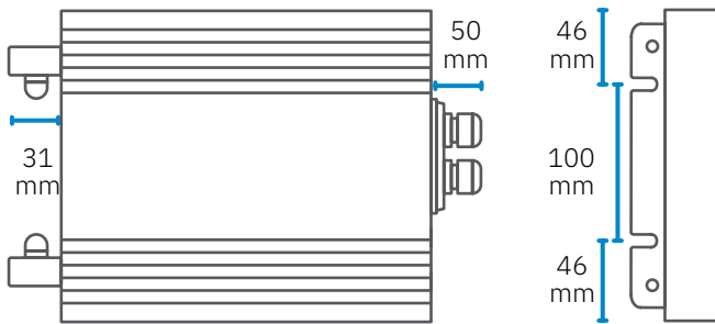
Vorstehende Anschlüsse
